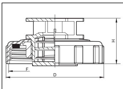
Крышка с дыхательным лабиринтным клапаном с прокладкой
