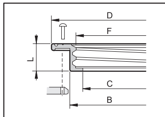
Резьбовое кольцо для бокового крепления
