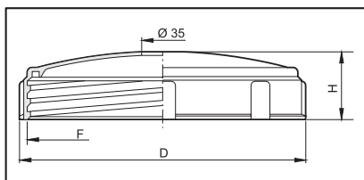
Крышка с отверстием для дыхательного клапана
