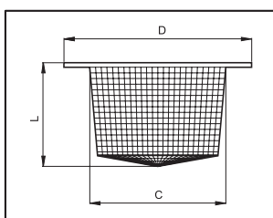
Полипропиленовый фильтр корзиночного типа
