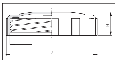
Прозрачная закрытая крышка с прокладкой
