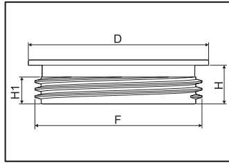
Закрытая крышка
