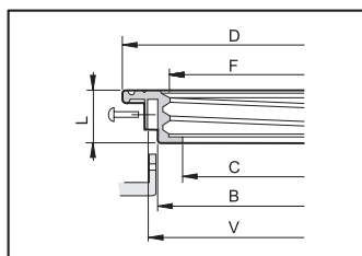
Уплотнительное кольцо между резервуаром и кольцом
