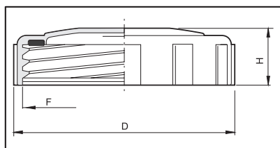
Закрытая крышка с прокладкой
