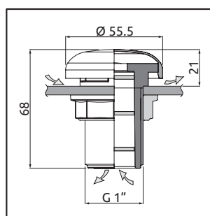
Лабиринтный дыхательный клапан
