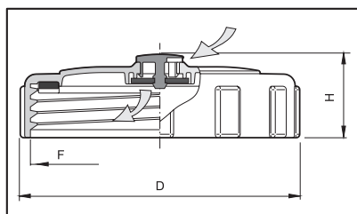
Крышка с мембранным дыхательным клапаном с прокладкой
