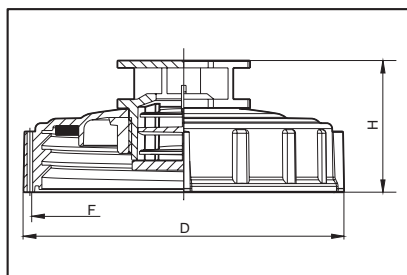
Крышка с дыхательным лабиринтным клапаном с прокладкой
