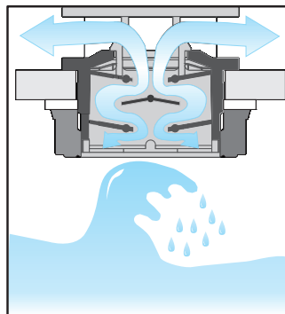
Pokrywa z zaworem odpowietrzającym labiryntowym i uszczelką
