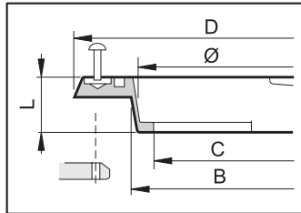
Резьбовое кольцо для плоских поверхностей
