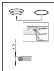
Уплотнительное кольцо между резервуаром и кольцом
