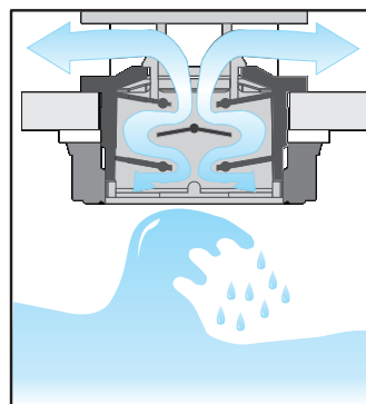
Крышка с дыхательным лабиринтным клапаном с прокладкой
