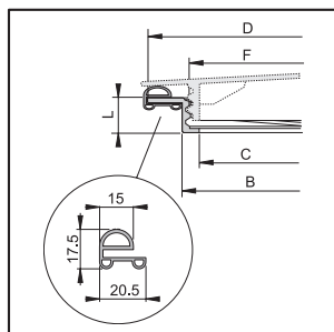
Резьбовое кольцо с двойной прокладкой для плоских поверхностей
