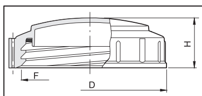
Закрытая крышка с прокладкой
