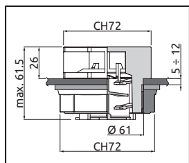
Entlüftungsventil mit Schwimmkugel
