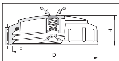
Закрытая крышка с прокладкой
