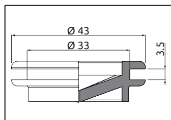
Лабиринтный дыхательный клапан
