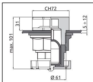
Поплавковый клапан
